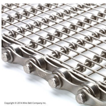
网带边缘带链条，空心销链式或链节式
